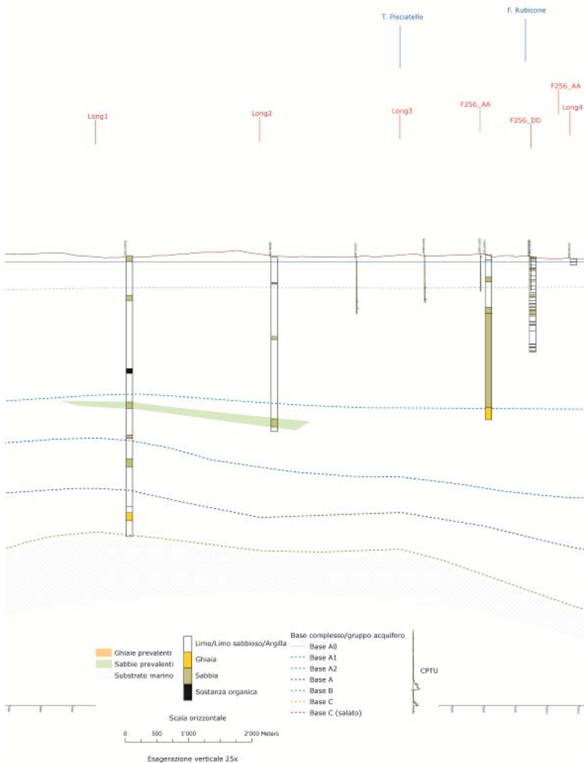
Figura n. 19 - Sezione 145 sviluppata parallelamente alla costa passante nei pressi di Borella Cervia (ID_el = 2).
