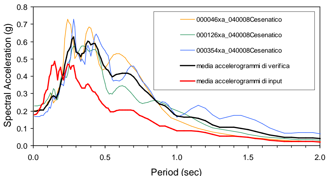
Figura n. 41 - Spettro di risposta in superficie.
