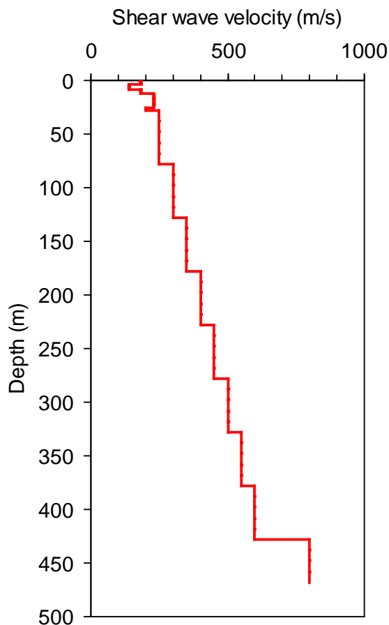
Figura n. 40 - Profilo di Vs di riferimento per le analisi di risposta sismica locale.
